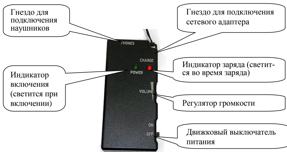
Рис. 6 Приемное устройство (ППМ)
